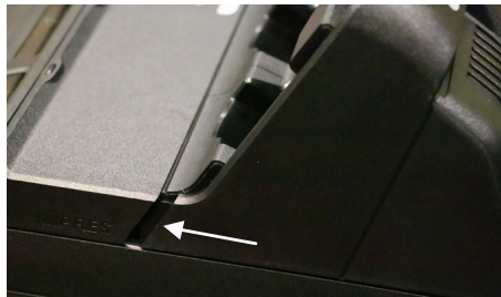
Figura 32: Instalação dos parafusos da tampa superior
