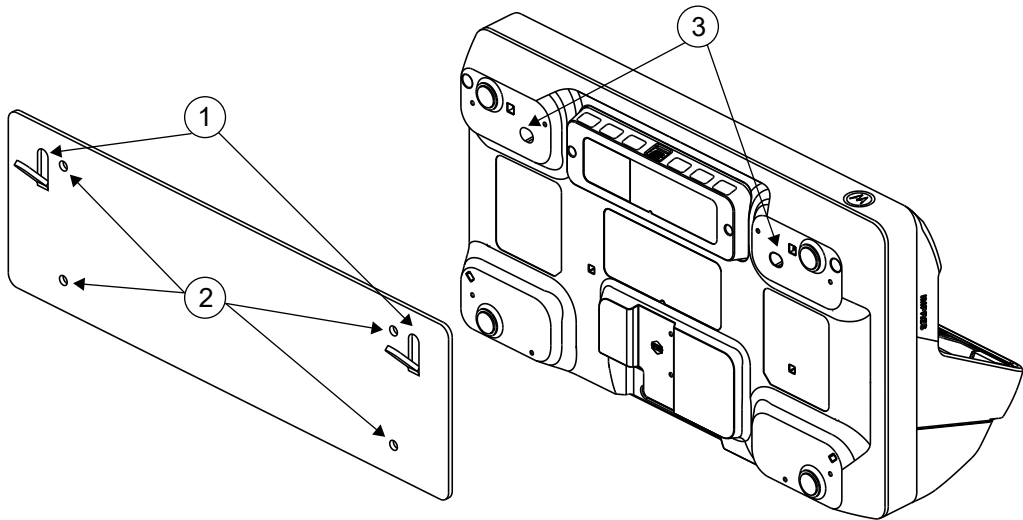
Figura 22: Orifícios de montagem do suporte e posição das travas
