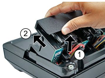
Figura 27: Remoção do encaixe do compartimento
