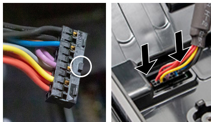
Figure 29 : Alignez et poussez le connecteur vers le bas dans le chargeur
